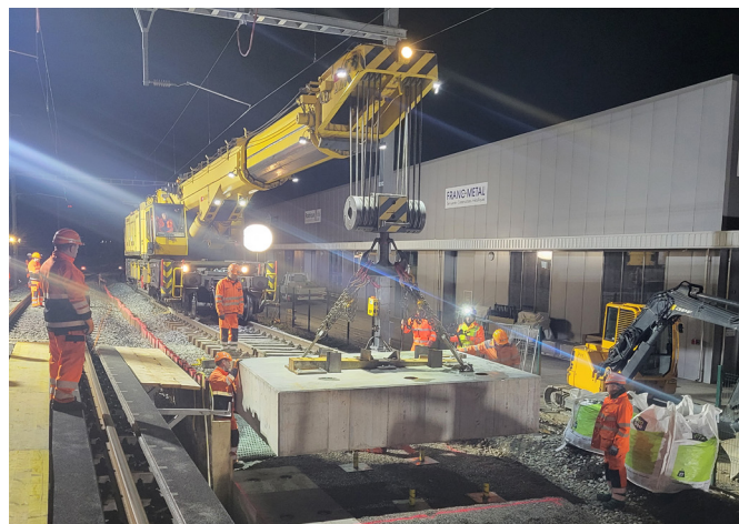
Mise en place des appuis pour les ponts provisoires
