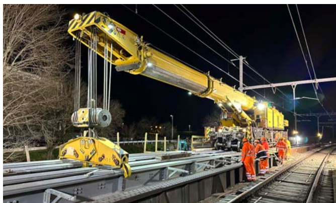
Source photo : Perret-Gentil SA > Pose des ponts provisoires
