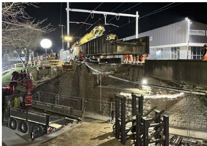
Source photo : Perret-Gentil SA > Dépose pont métallique 47 tonnes existant
